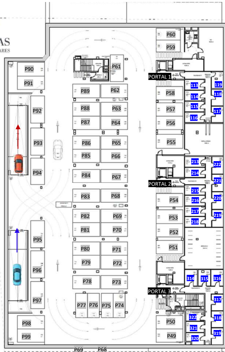
SÓTANO 2
