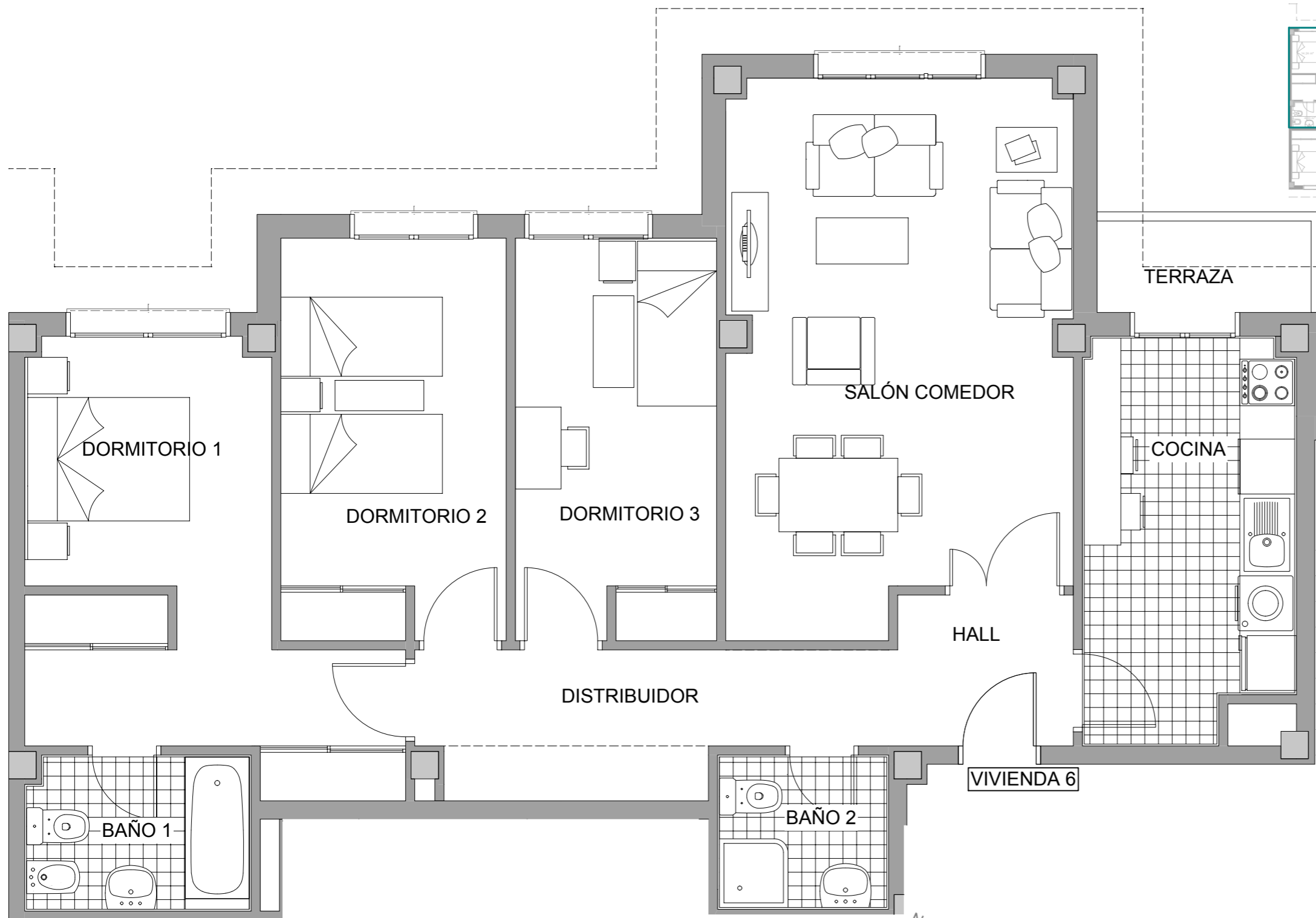
VIVIENDA 6. ESCALERA 3Y4 PLANTA PRIMERA Y SEGUNDA
